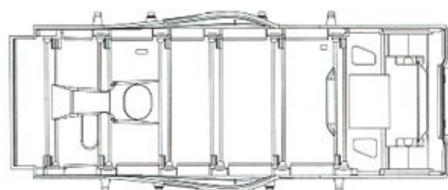
HULL 车体
