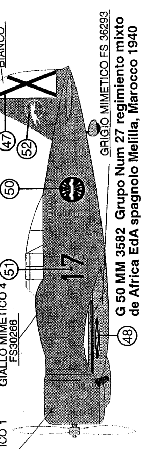
VERDE MIMETICO 1 FS.34258 GIALLO MIMETICO 4 FS.30266 BRUNO MIMETICO 10 FS.30045 GRIGIO MIMETICO FS.36293 G 50 Bis - 150° Sq. Libia Giugno 1941 Cap. Tullio De PRATO
