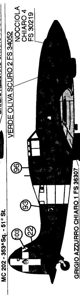
VERDE OLIVA SCURO 2 FS 34052 NOCCIOLA CHIARO 4 FS 30219 MC 202 - 353 a Sq. - 51 o St. GRIGIO AZZURRO CHIARO 1 FS 36307
