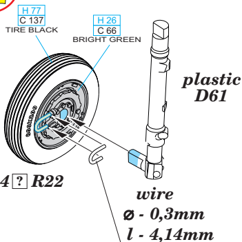
wire Ø - 0,3mm l - 4,14mm
