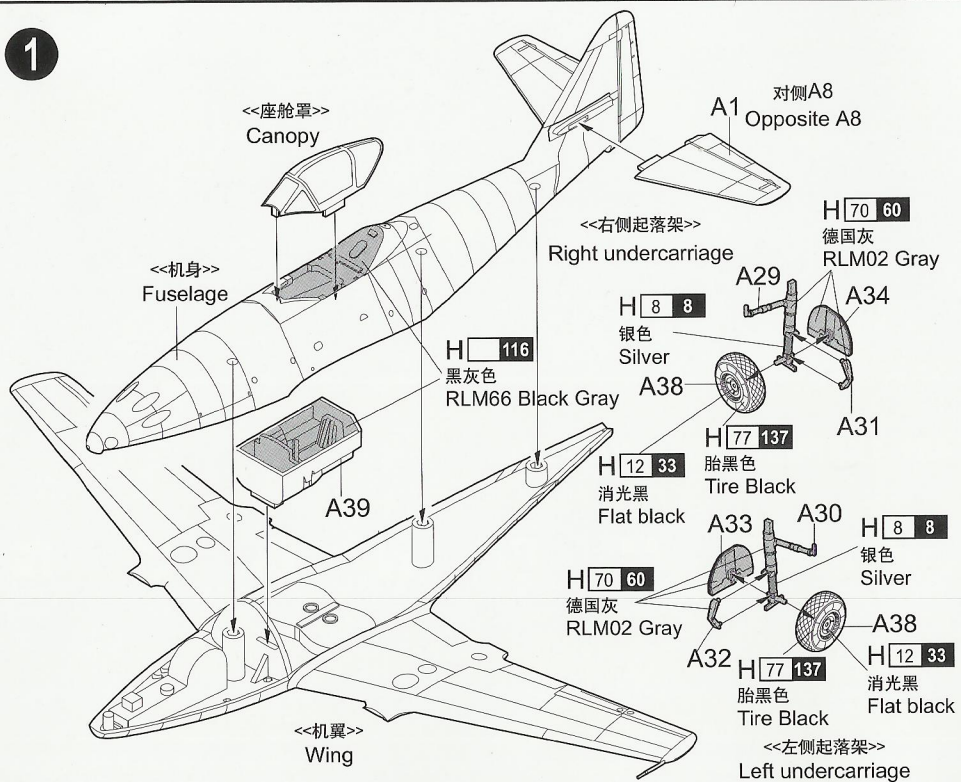
部品图 Parts
