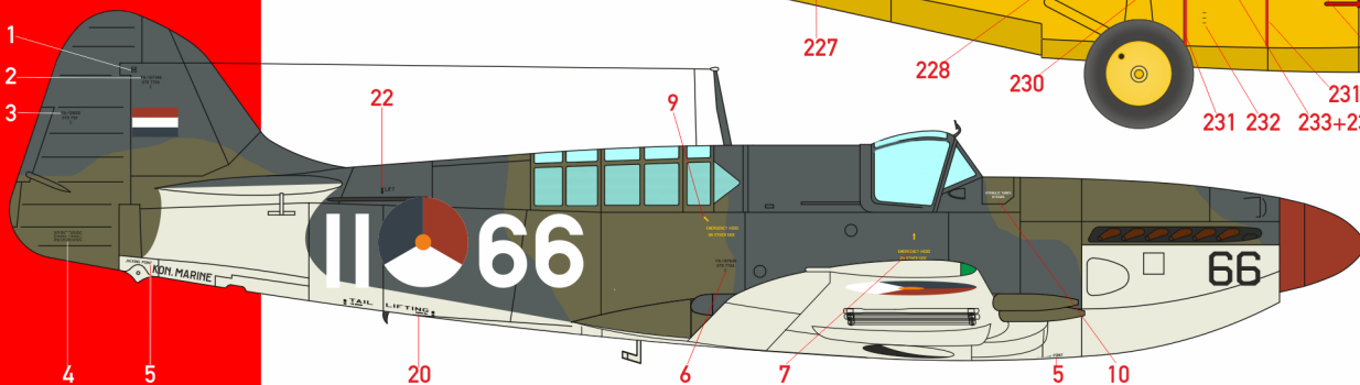
Fairey Firefly F.Mk.IV, K66, VSQ 1, Hr.Ms. Karel Doorman, 1e Westreis, West-Indië, Hato, Curaçao, Februari 1950.
