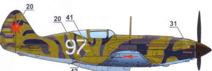
7) МиГ-3 "Білий 97", 55й ВАП ВПС СРСР, 1941р. "White 97", 55th Fighter reg. Soviet AF, 1941.
