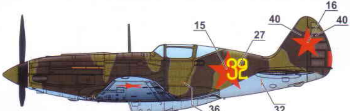
2) МиГ-3 "Жовтий 32", захоплений німецькими військами, літо 1941р. "Yellow 32", captured by German forces, Summer 1941.
