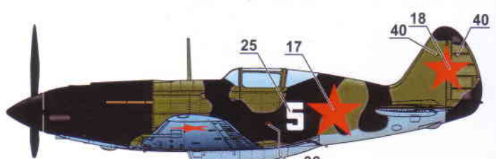
14) МиГ-3 "Білий 5", 8й ВАП ЧФ СРСР, 1942р. "White 5", 8th Fighter reg., Black Sea fleet, 1942.
